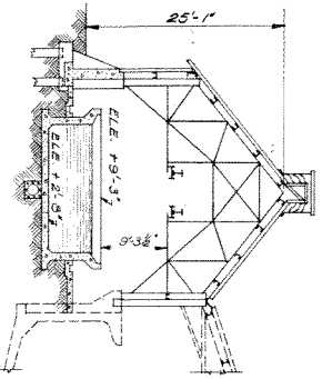
SECTION D-D SCALE: \frac{1}{8}'' = 1'-0''
