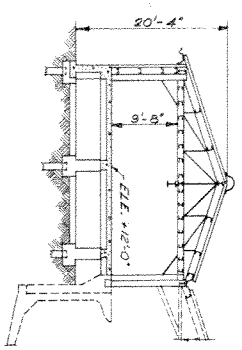
SECTION B-B SCALE: \frac{1}{8}'' = 1'-0''
