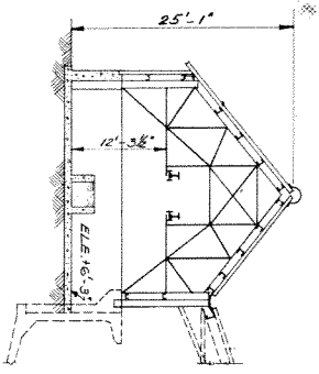
SECTION C-C SCALE: \frac{1}{8}'' = 1'-0''
